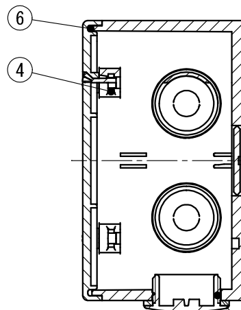
断面 A-A
